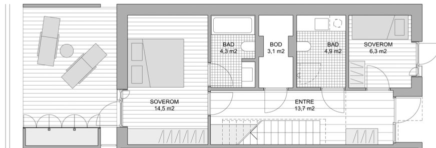
PLAN 1. ETASJE
