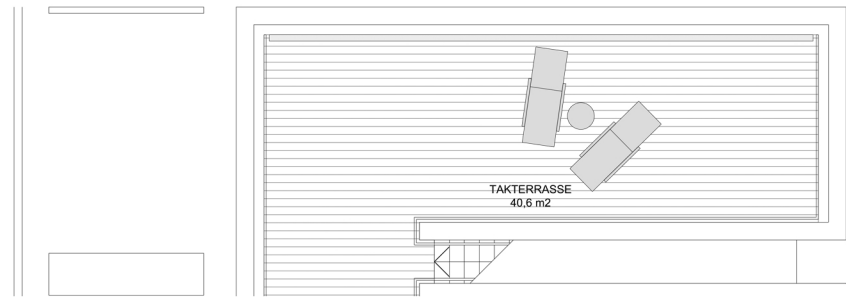
PLAN 3. ETASJE
